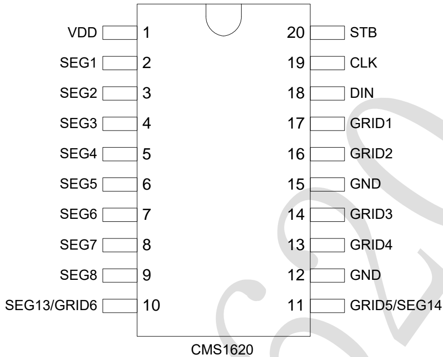
CMS1620 引脚说明:
