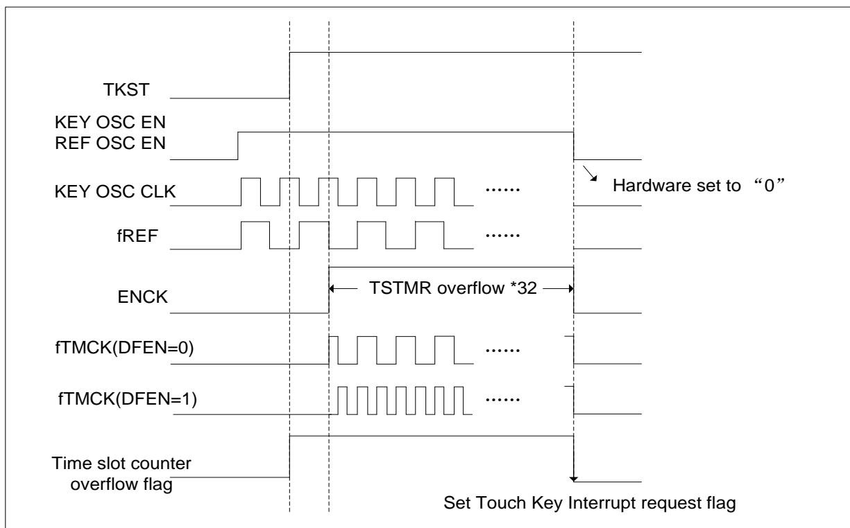
图 14-3: 触摸按键感应振荡器和参考振荡器时序方框图
