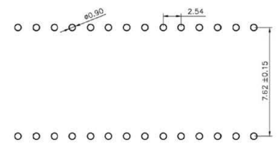
P.C.B LAYOUT
