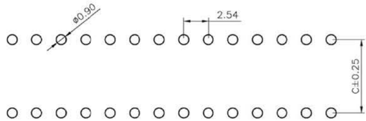
P.C.B LAYOUT
