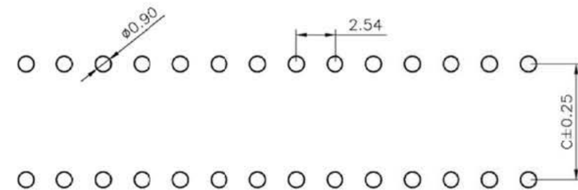
P.C.B LAYOUT
