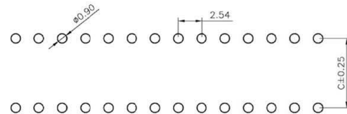
P.C.B LAYOUT
