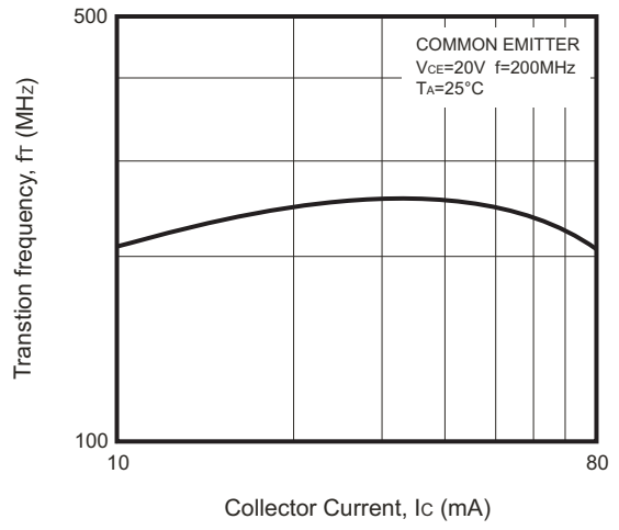
Fig.7 - F_T — I_c
