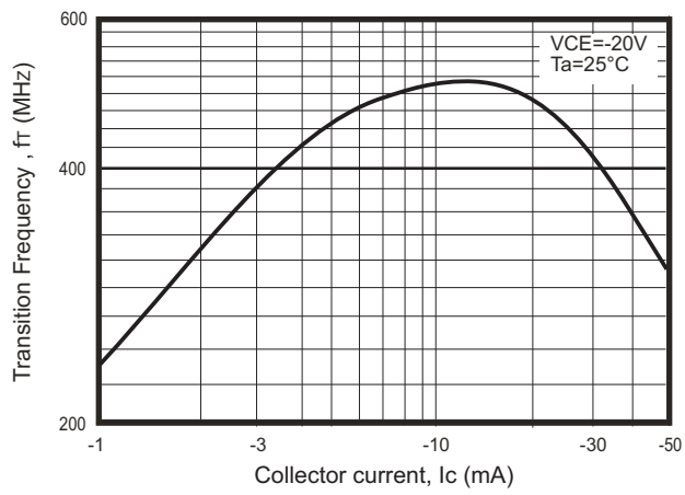
Fig.7 - f_T — I_C
