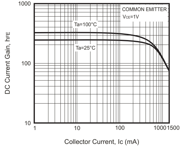
Fig.2 - h_{FE} - I_c
