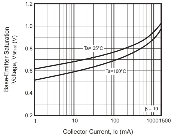
Fig.4 - V_{BEsat} - I_c
