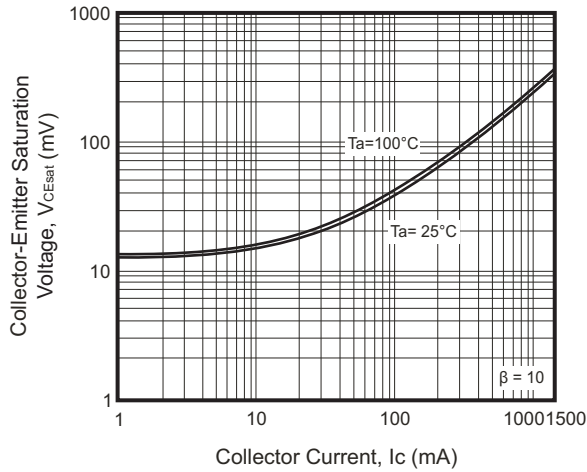
Fig.3 - V_{CEsat} - I_c
