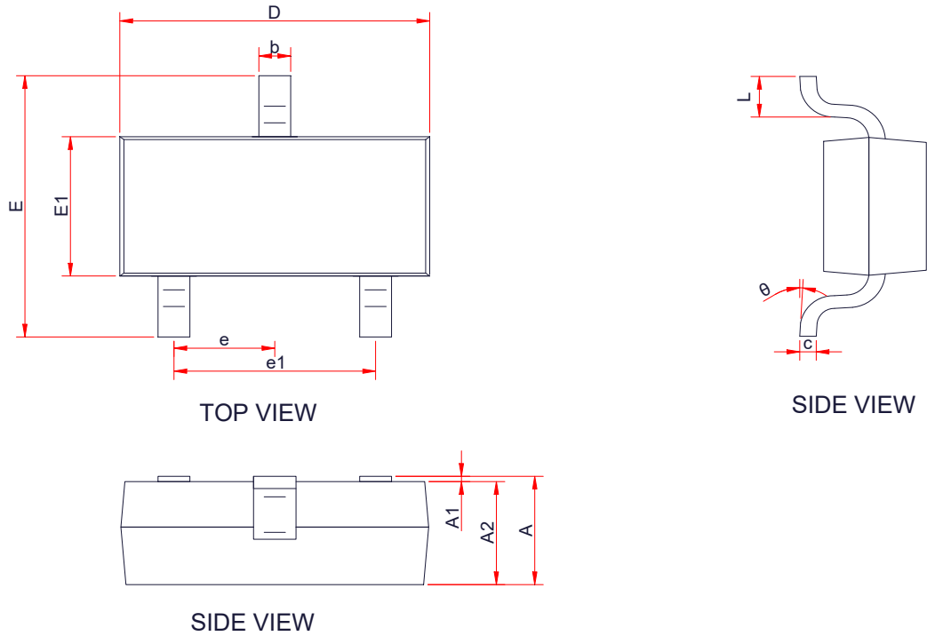
SOT-23-3L
