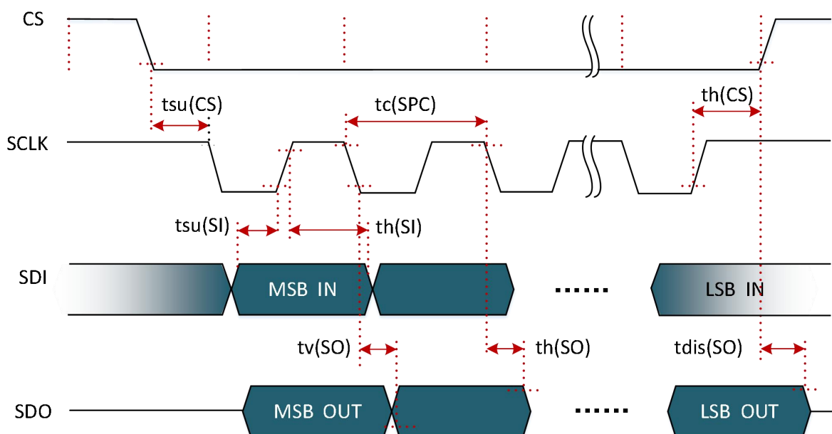
图 12-1 SPI 时序图
