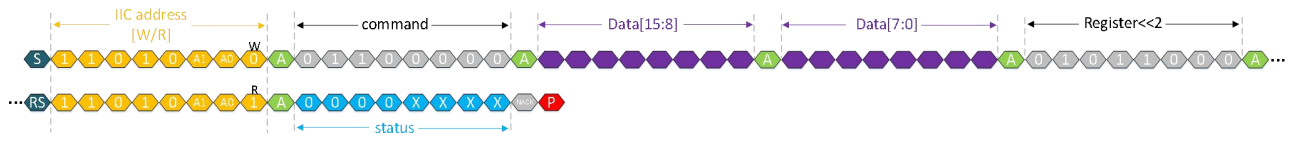
图 15-8. 写寄存器 0x16 I2C 时序图
