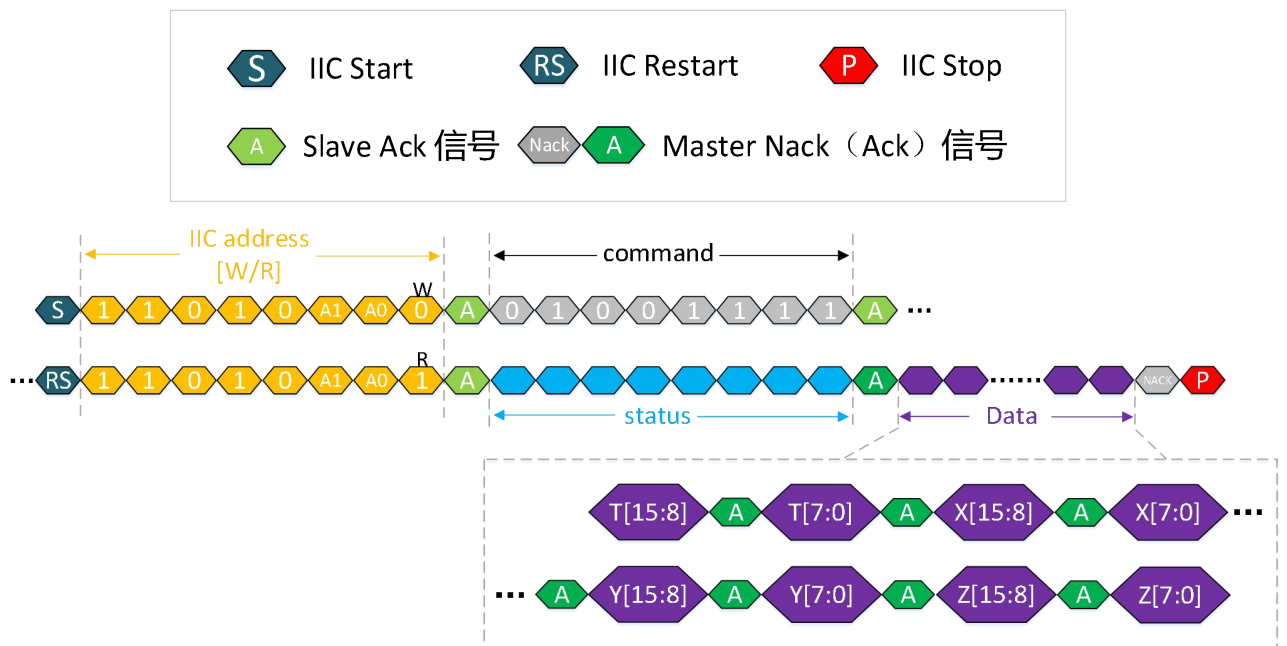
图 11-6. TXYZ 方式 data 回读 I2C 通信示意图
