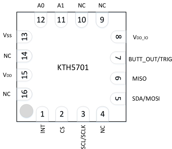
图 5-1.QFN3x3 16-Pin 顶视图
