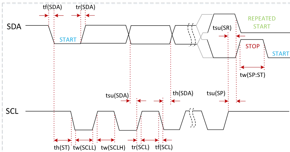
图 9-2 I2C 时序图
