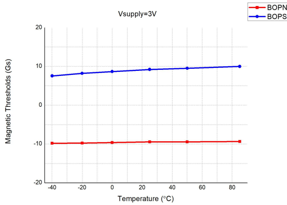
磁场阈值 vs 温度 @VDD=3.0V
