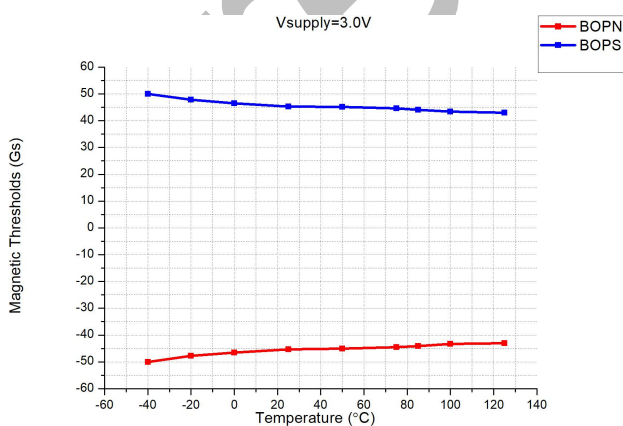
磁场阈值 vs 温度 @VDD=3.0V
