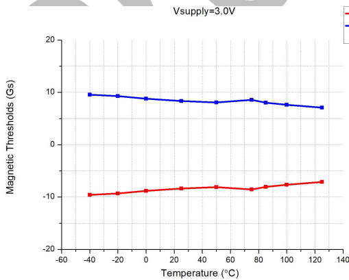
磁场阈值 vs 温度 @VDD=3.0V
