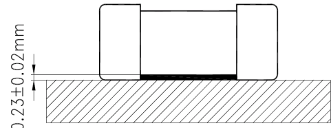
建議點膠位置示意圖
