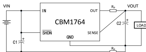
图 1 开尔文检测连接方式
