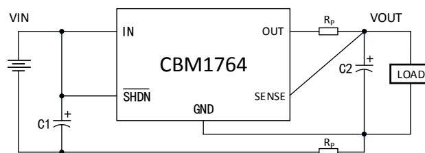
图 1 开尔文检测连接方式
