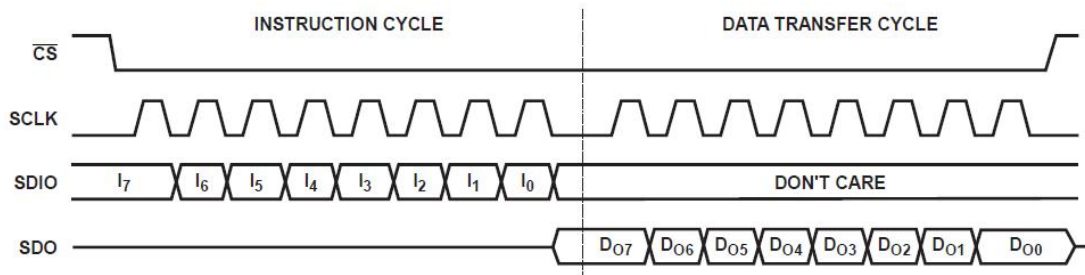
图 15 三线式串行端口读取时序—时钟空闲为低
