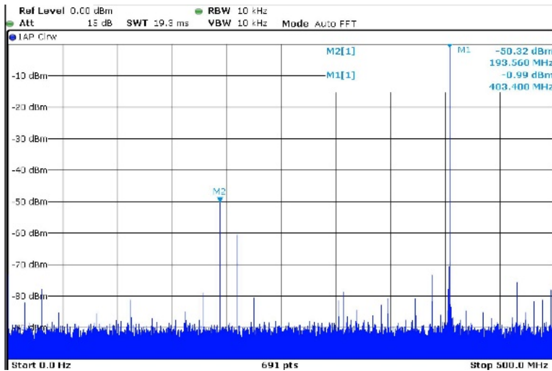
图 5 403.1MHz 条件下的宽带 SFDR , REFCLK=1GHZ
