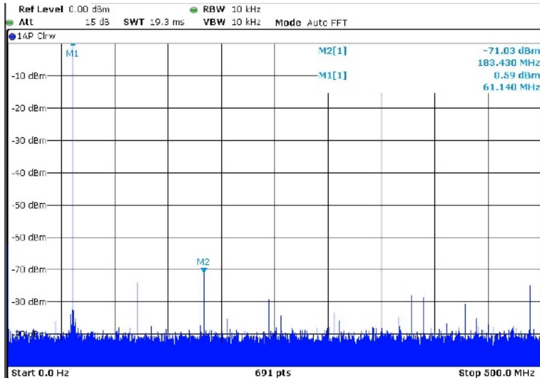
图 3 61.1MHz 条件下的宽带 SFDR , REFCLK=1GHZ
