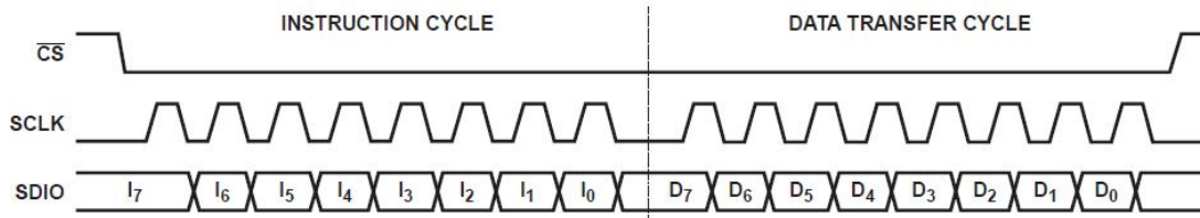
图 14 串行端口写入时序—时钟空闲为低
