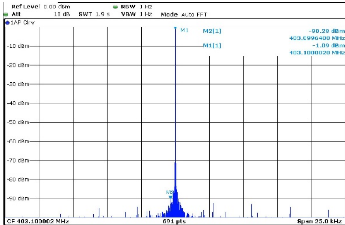
图 8 图 5 的窄带视图 (带有载波和下边带抑制)
