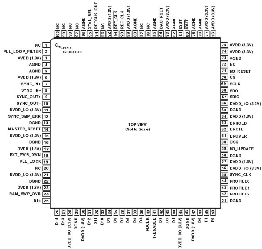
图 2 芯片管脚图
