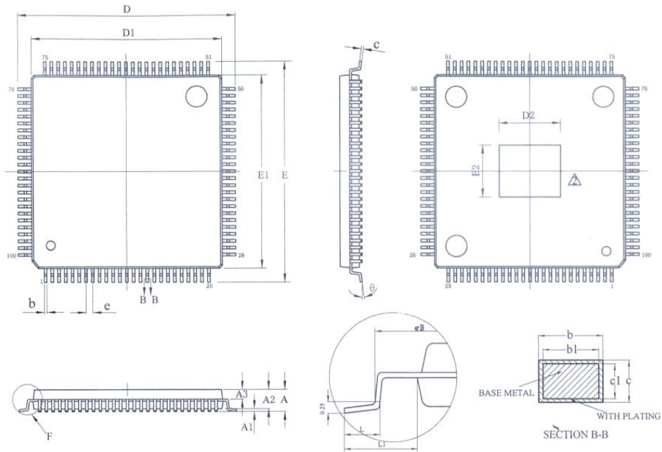
100 引脚裸露焊盘、超薄四方扁平封装[TQFP_EP](SV-100-4)尺寸(单位:mm)
