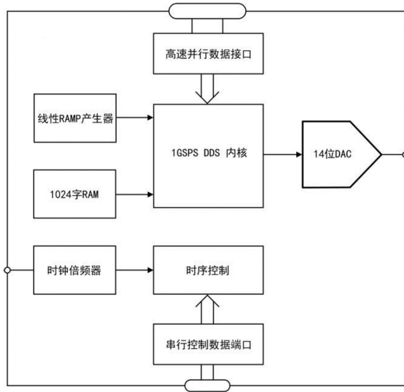
图 1 CBM99D10 功能框图
