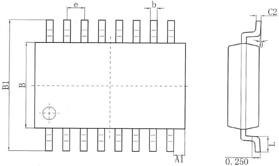
图 2: 封装尺寸图
