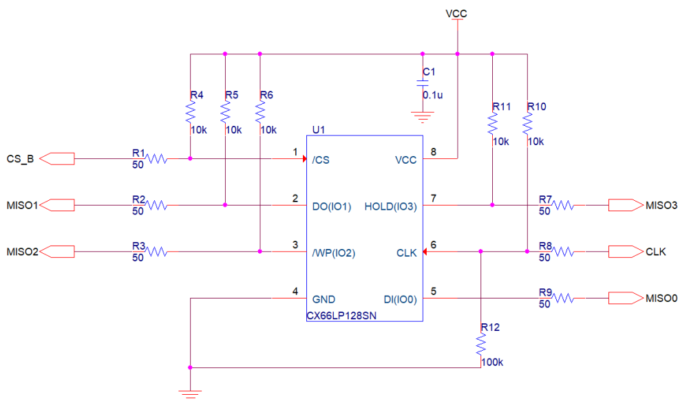
图 14 典型应用
