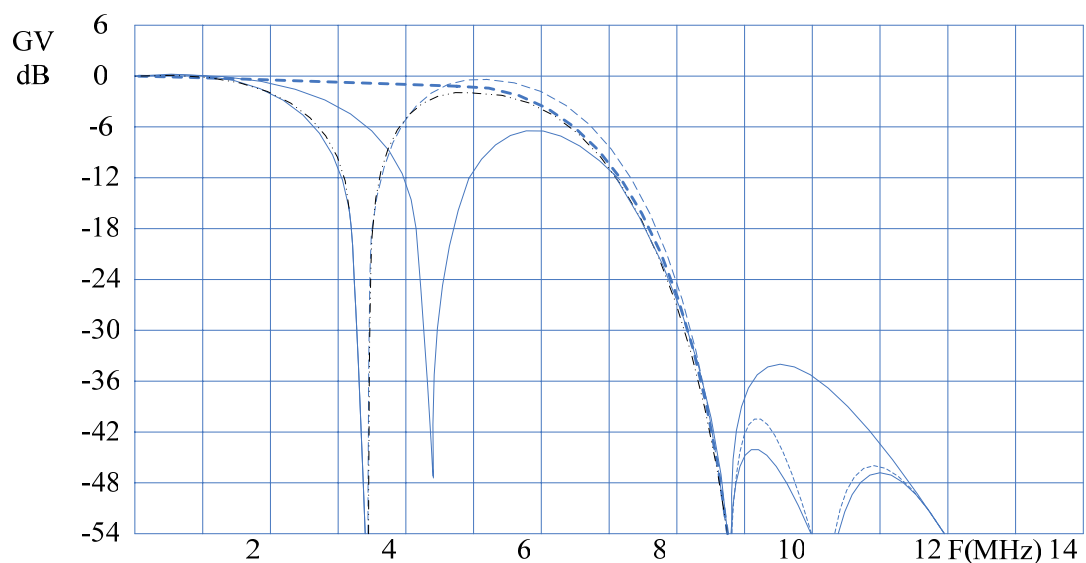
图 2 亮度滤波器频谱图
