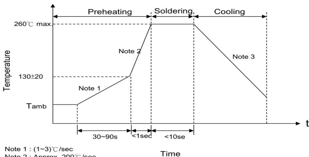
(图 2: 波峰焊曲线图)
