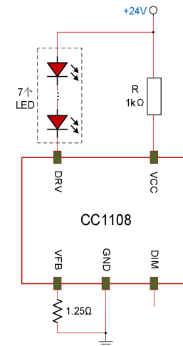
典型 24V 120mA 应用电路
