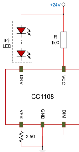
典型 24V 60mA 应用电路
