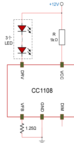
典型 12V 120mA 应用电路
