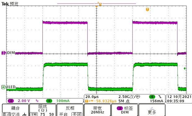
DIM & ILED 波形 (常温, DIM 为 50% 占空比)
