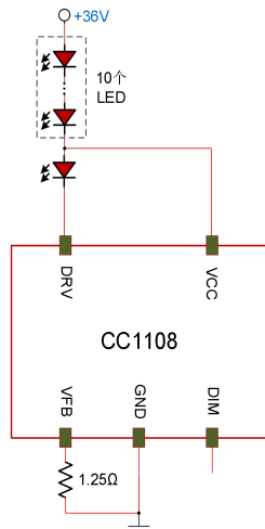
典型 36V 120mA 应用电路
