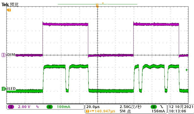
DIM & ILED 波形 (高温, DIM 为 50% 占空比)
