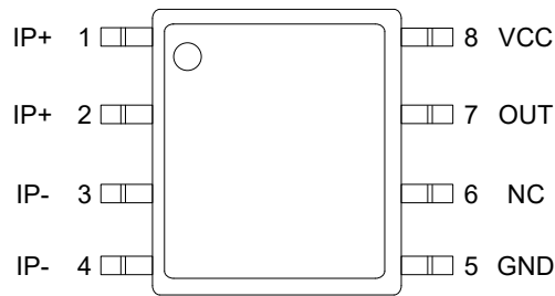
SOP8 封装
