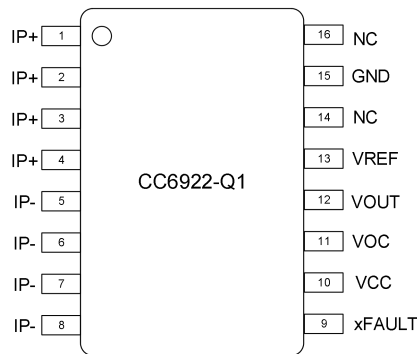
SOP16W 封装
