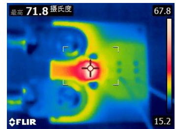
封装体热成像图（输入电流 60A）
