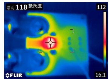
封装体热成像图（输入电流 80A）
