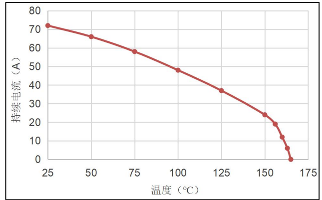
持续电流 I CON vs 温度
