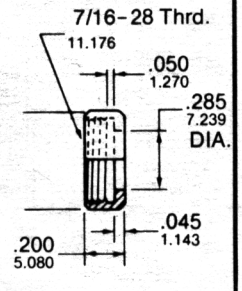
1/2" HEX NUT
