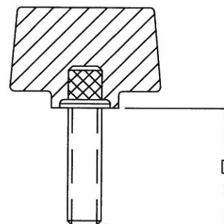
THREADED STUD
