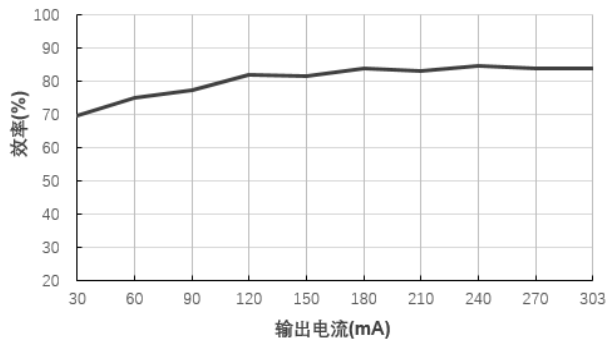
效率Vs输出电流(Vin=24V)@B2403LS-1WR3
