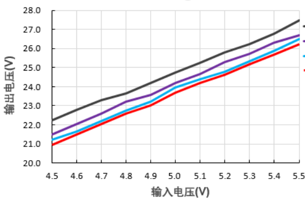
输出电压Vs输入电压@B0524LS-1WR3
