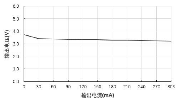
输出电压 VS 输出电流 (B1203S-1W@Vin=12V)
