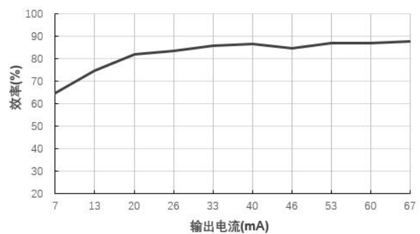
效率 VS 输出电流 (B0515S-1W@Vin=5V)
