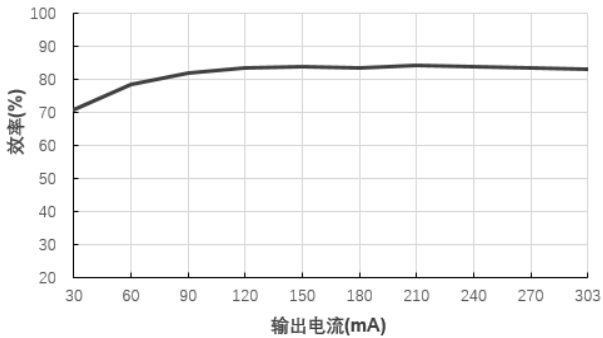
效率Vs输出电流(Vin=5V)@B0503LS-1WR2
