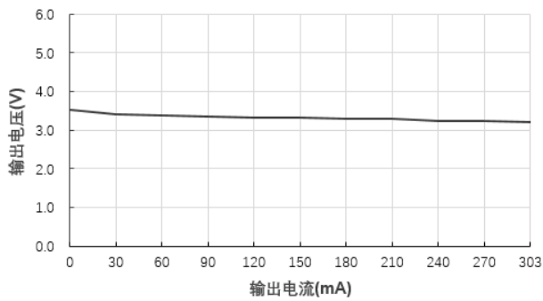
输出电压Vs输出电流(Vin=5V)@B0503LS-1WR2
