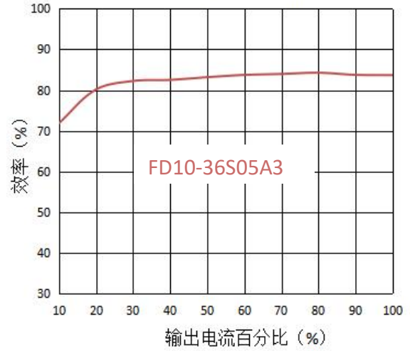
输出效率vs输出负载 (48V输入)
