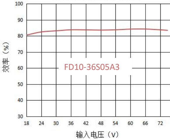
输出效率vs输入电压 (满载)
