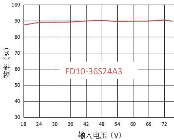
输出效率vs输入电压 (满载)
