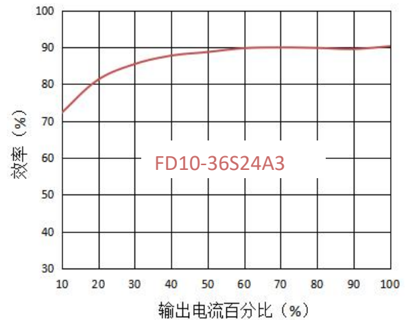
输出效率vs输出负载 (48V输入)
