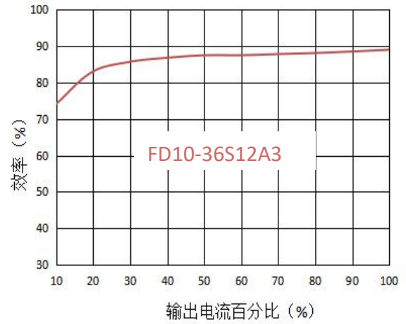
出效率vs输出负载 (48V输入)
