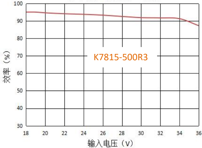
输出效率vs输入电压 (满载)
