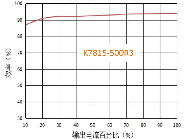
输出效率vs输出负载 (24V输入)
