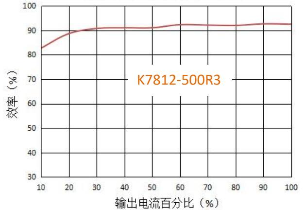
输出效率vs输出负载 (24V输入)
