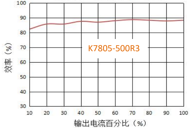
输出效率vs输出负载 (24V输入)
