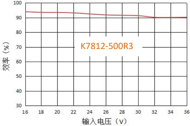
输出效率vs输入电压 (满载)
