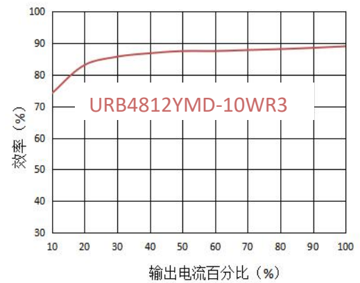
出效率vs输出负载 (48V输入)
