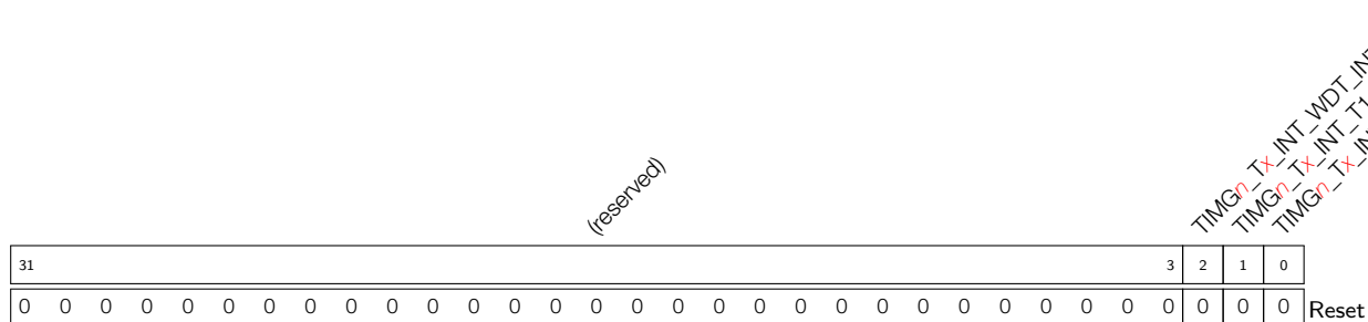
Register 18.22: TIMG n _Tx_INT_ST_REG (0x00a0)
