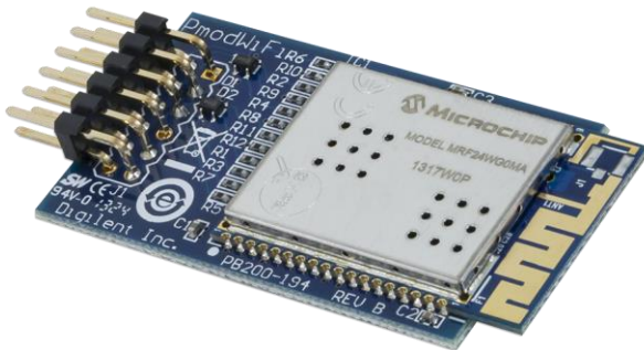
The PmodWiFi.
