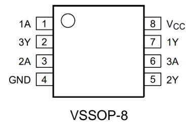
SSOP-8
