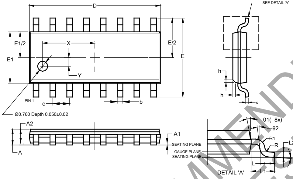
SO-16
