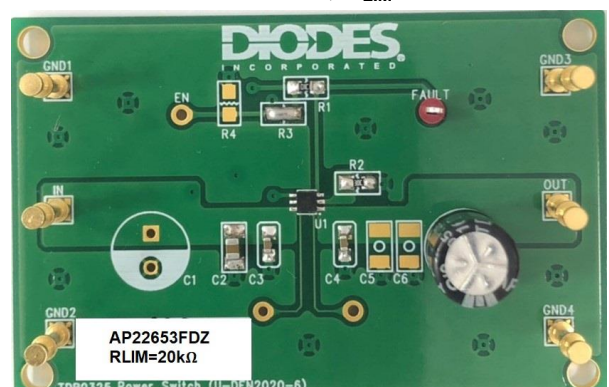
AP22653FDZ, R_{LIM}=20\text{k}\Omega
