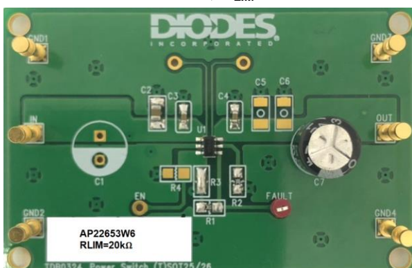
AP22653W6, R_{LIM}=20\text{k}\Omega
