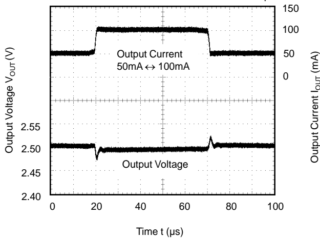
AP7315-25 V_{IN}=3.5\text{V} tr=tf=0.5\mu\text{s}
