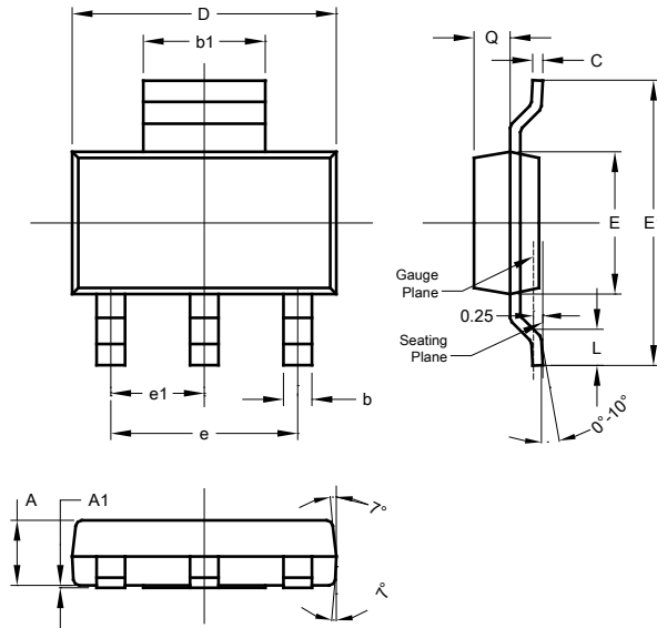
SOT223
