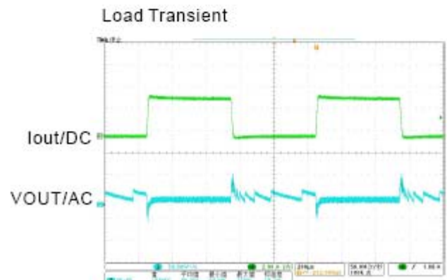
V_{in}=3.3\text{V} , V_o=1.2\text{V} , I_o=0\text{A}\sim 3.5\text{A} , f=1\text{kHz}
