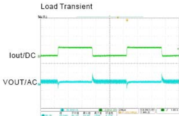
V_{in}=3.3\text{V} , V_o=1.2\text{V} , I_o=0.2\text{A}\sim 2\text{A} , f=1\text{kHz}
