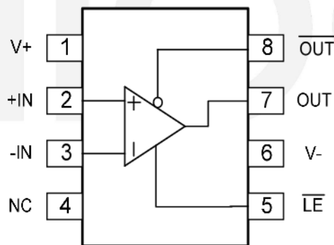
SOIC-8/MSOP-8
