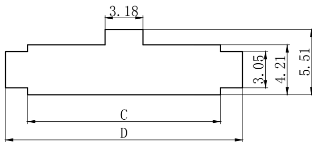
安装尺寸
