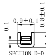
SECTION D-D
