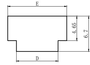
安装尺寸图
