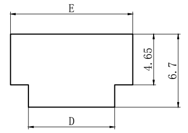
安装尺寸图
