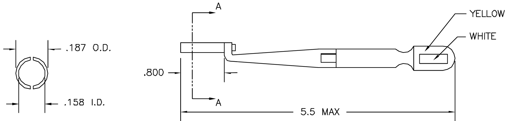
VIEW A-A
