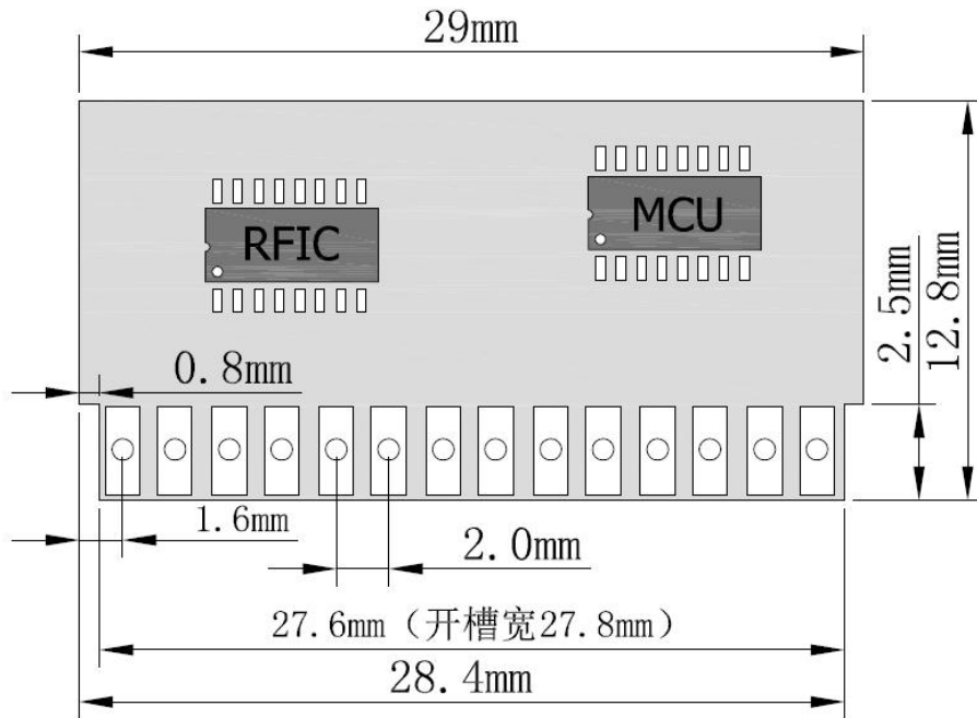
图 4 DL-RX06C-LO6 尺寸图
