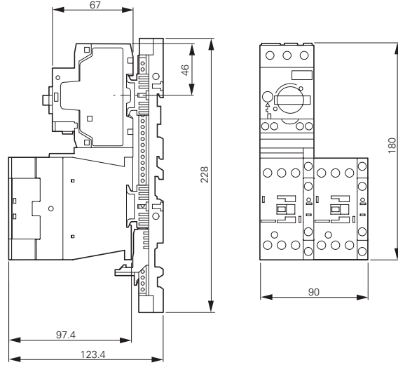
MSC-R-...-M17[...32]BBA...
